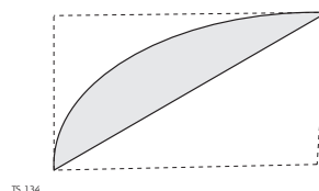
Сегмент
