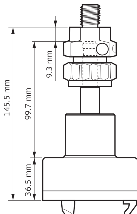
Трегер GRT247, предпочтителен для установки GS15 — корот. штатив
