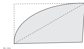
Сектор
