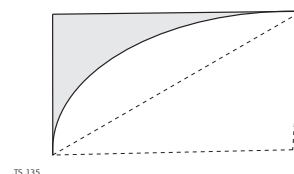
Площадь скругления
